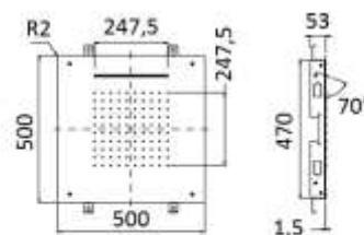
DESENHO DIMENSIONAL | DIMENSIONAL DRAWING
