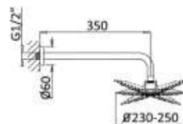
DESENHO DIMENSIONAL | DIMENSIONAL DRAWING
