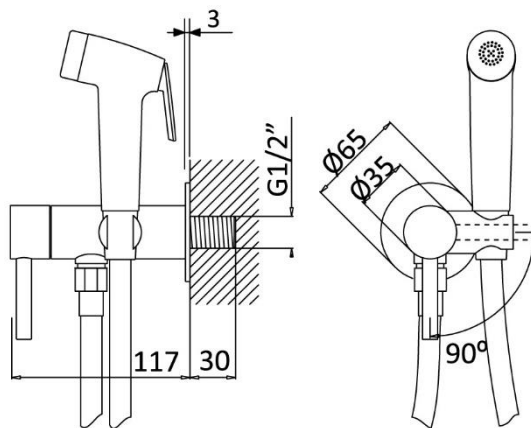
DESENHO DIMENSIONAL | DIMENSIONAL DRAWING
