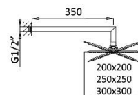
DESENHO DIMENSIONAL | DIMENSIONAL DRAWING
